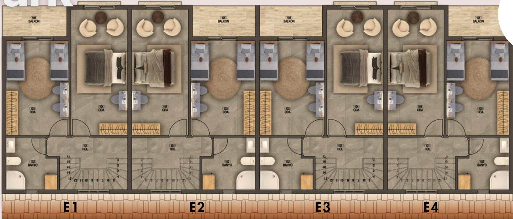
E BLOK 1. KAT PLANI
