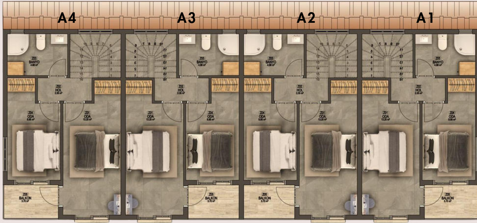
A BLOK 1.KAT PLANI
